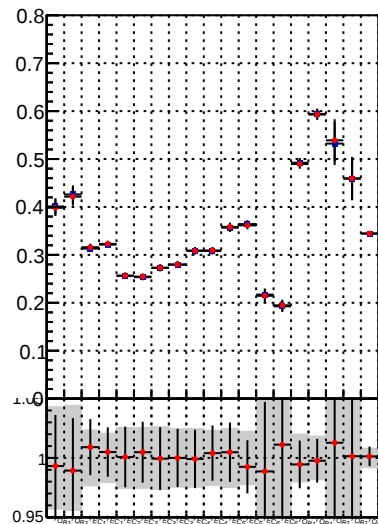
Fake rate vs. —●— DQM TT mkFit-DQM_original —●— DQM TT mkFit-DQM_modified5
