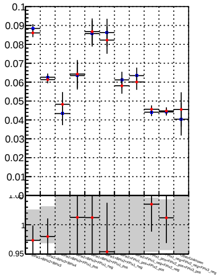
Fake rate vs. DQM TT mkFit-DQM_original DQM TT mkFit-DQM_modified5
