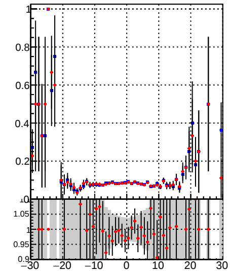
—■— DQM\_TT\_mkFit-DQM\_original —●— DQM\_TT\_mkFit-DQM\_modified5
