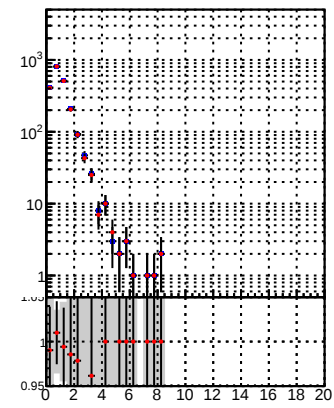
N of reco track vs. \chi^2 DQM TT mkFit-DQM_original DQM TT mkFit-DQM_modified5
