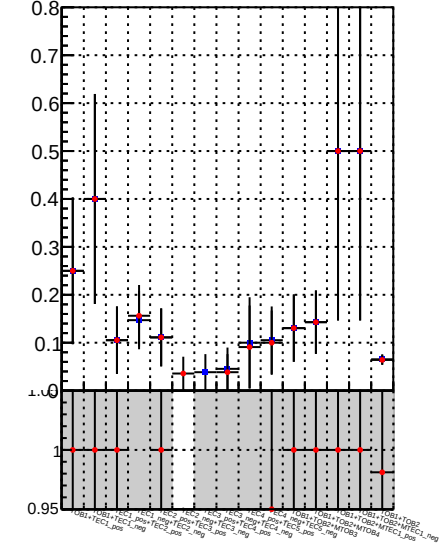
Fake rate vs. DQM TT mkFit-DQM_original DQM TT mkFit-DQM_modified5
