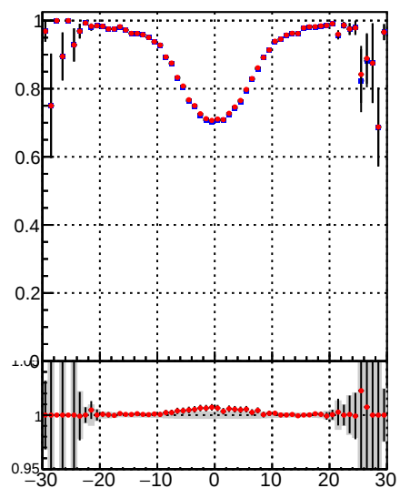
—●— DQM TT mkFit-DQM_original —●— DQM TT mkFit-DQM_modified5
