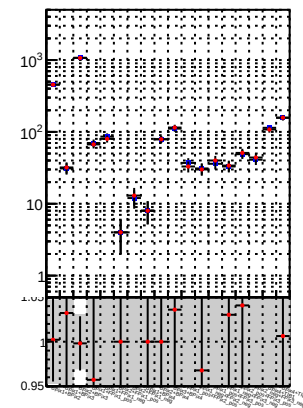
N of reco track vs. \chi^2 DQM TT mkFit-DQM_original DQM TT mkFit-DQM_modified5
