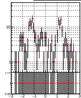
█ DQM_TT_mkFit-DQM_original █ DQM_TT_mkFit-DQM_modified5
