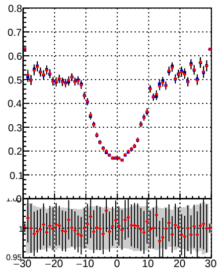
—●— DQM\_TT\_mkFit-DQM\_original —●— DQM\_TT\_mkFit-DQM\_modified5
