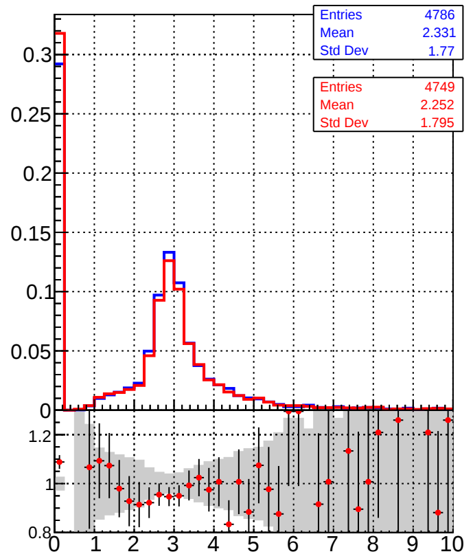
dE/dx estimator 2
