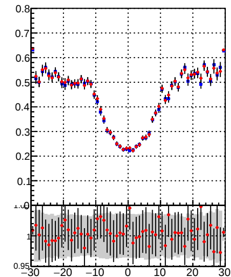
—●— DQM\_TT\_mkFit-DQM\_original —●— DQM\_TT\_mkFit-DQM\_modified4
