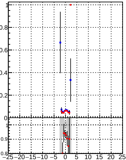
—●— DQM\_TT\_mkFit-DQM\_original —●— DQM\_TT\_mkFit-DQM\_modified3
