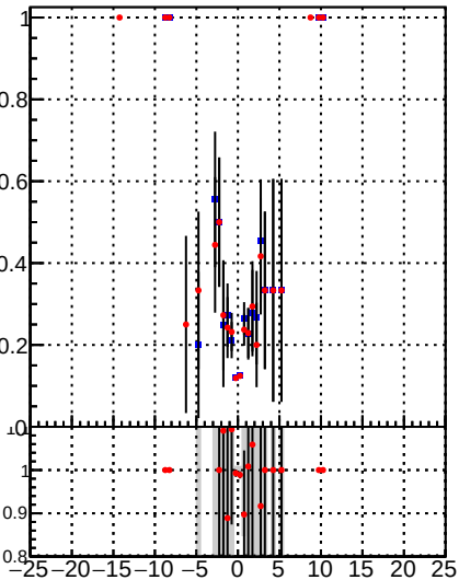
—●— DQM TT mkFit-DQM_original —●— DQM TT mkFit-DQM_modified3
