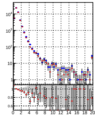
Legend: DQM TT mkFit-DQM_original DQM TT mkFit-DQM_modified3
