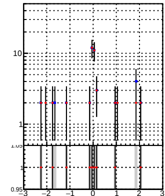
pT eta
