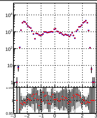
—●— DQM TT mkFit-DQM_original —●— DQM TT mkFit-DQM_modified3
