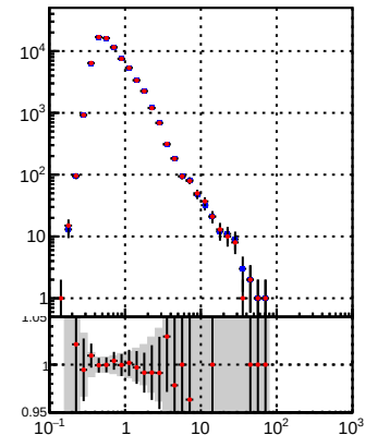
—●— DQM TT mkFit-DQM_original —●— DQM TT mkFit-DQM_modified3
