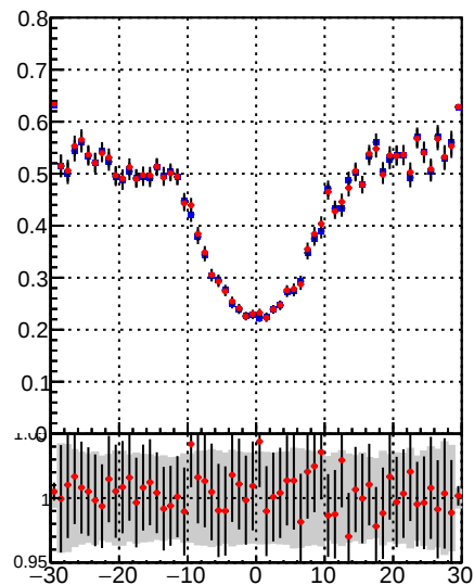
—•— DQM\_TT\_mkFit-DQM\_original —•— DQM\_TT\_mkFit-DQM\_modified3
