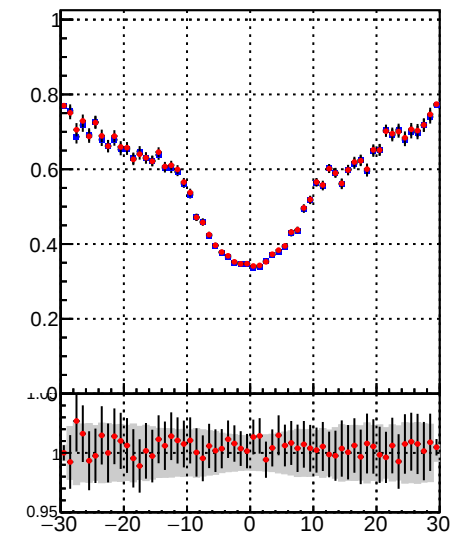
—◆— DQM\_TT\_mkFit-DQM\_original —◆— DQM\_TT\_mkFit-DQM\_modified3
