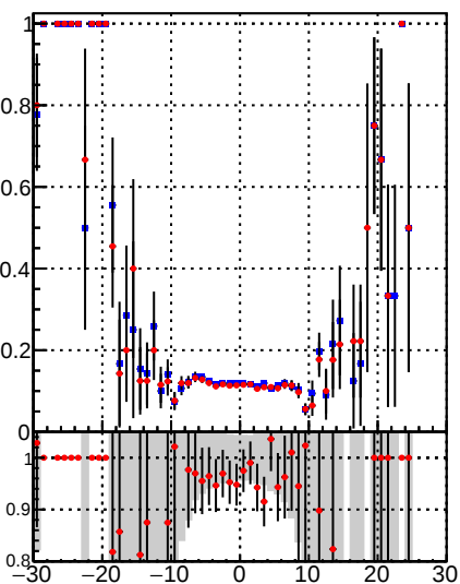
Fake rate vs d —●— DQM TT mkFit-DQM_original —●— DQM TT mkFit-DQM_modified3
