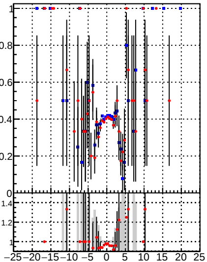
—●— DQM TT mkFit-DQM_original —●— DQM TT mkFit-DQM_modified3
