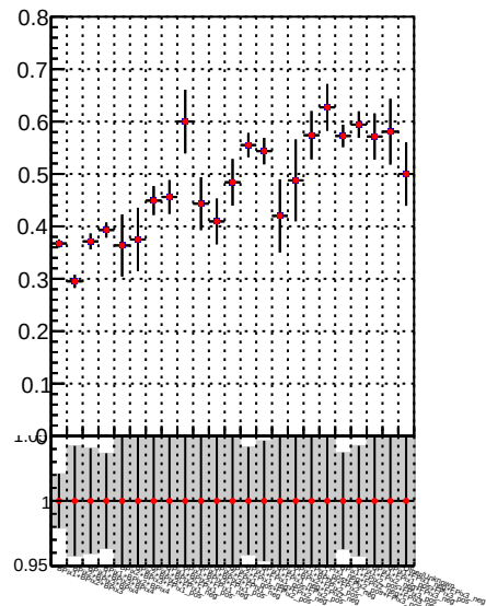
Fake rate vs. DQM TT mkFit-DQM_original DQM TT mkFit-DQM_modified2
