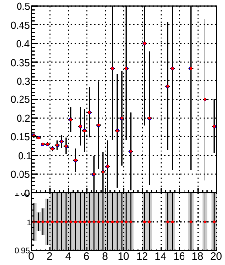
Fake rate vs. \chi^2 DQM TT mkFit-DQM_original \chi^2 DQM TT mkFit-DQM_modified2
