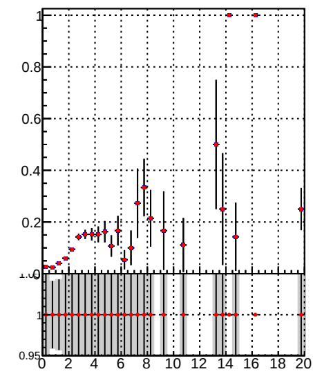
Fake rate vs. \chi^2 DQM TT mkFit-DQM_original \chi^2 DQM TT mkFit-DQM_modified2
