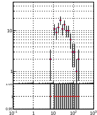
—●— DQM TT mkFit-DQM original —●— DQM TT mkFit-DQM modified2
