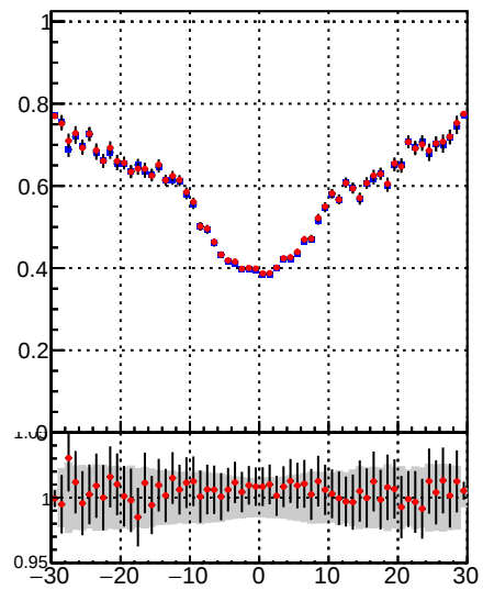
—◆— DQM\_TT\_mkFit-DQM\_original —◆— DQM\_TT\_mkFit-DQM\_modified
