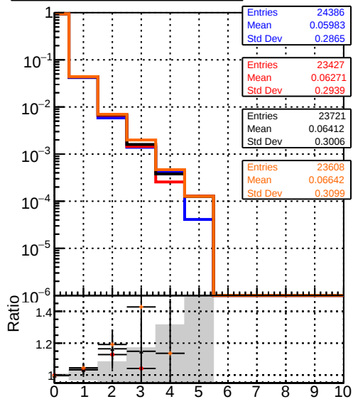
mean hit — DQM_mkFit_newBASE3 — DQM_mkFit_new — DQM_mkFit_newANDPL — DQM_mkFit_newiOKKK
