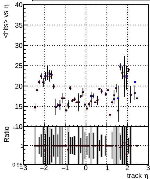
mean hits — DQM_TT_CKF_ORIG — DQM_TT_CKFandPless_ORIG — DQM_TT_CKFandPless_MODIF
