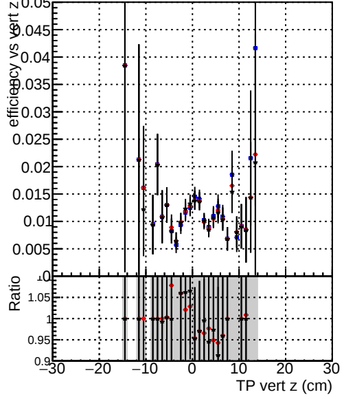
Efficiency vs. TP vert z —●— DQM_TT_CKF_ORIG —●— DQM_TT_CKFandPless_ORIG —●— DQM_TT_CKFandPless_MODIF
