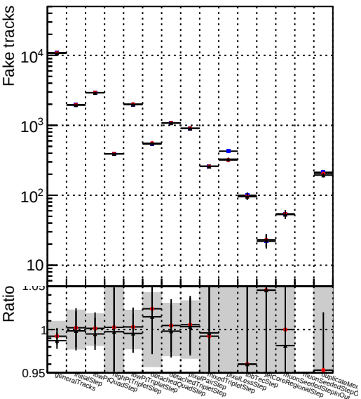
DQM_TT_CKFandPless_ORIG DQM_TT_CKFandPless_MODIF
