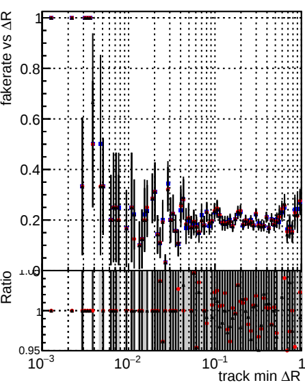
Fake rate vs \Delta R(\text{track, jet}) Legend: DQM_TT CKF_ORIG DQM_TT CKFandPless_ORIG DQM_TT CKFandPless_MODIF
