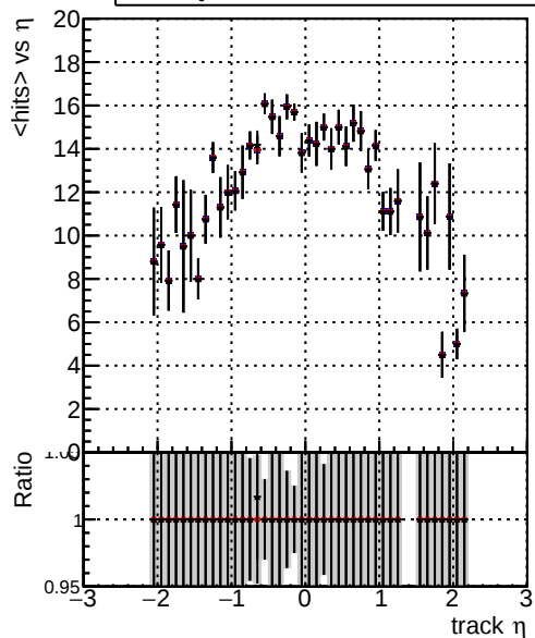
mean hit — DQM_TT_CKF_ORIG — DQM_TT_CKFandPless_ORIG — DQM_TT_CKFandPless_MODIF
