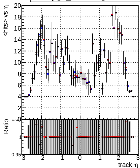
mean hit — DQM_TT_CKF_ORIG — DQM_TT_CKFandPLess_ORIG — DQM_TT_CKFandPLess_MODIF
