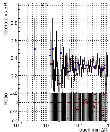
—•— DQM TT CKF ORIG —•— DQM TT CKFandPless ORIG —•— DQM TT CKFandPless MODIF
