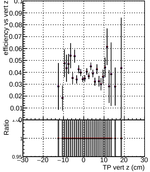
Efficiency vs. TP vert z (cm) — DQM_TT_CKF_ORIG — DQM_TT_CKFandPLess_ORIG — DQM_TT_CKFandPLess_MODIF
