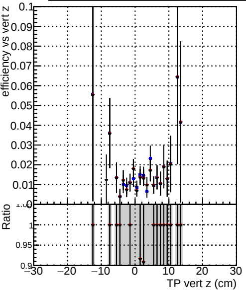
Efficiency vs vertpos DQM_TT_CKF_ORIG DQM_TT_CKFandPLess_ORIG DQM_TT_CKFandPLess_MODIF
