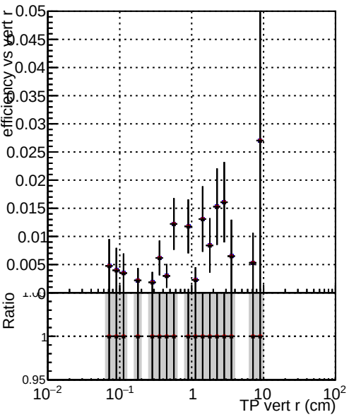
Efficiency vs TP vert r (cm) Legend: DQM_TT_CKF_ORIG DQM_TT_CKFandPLess_ORIG DQM_TT_CKFandPLess_MODIF
