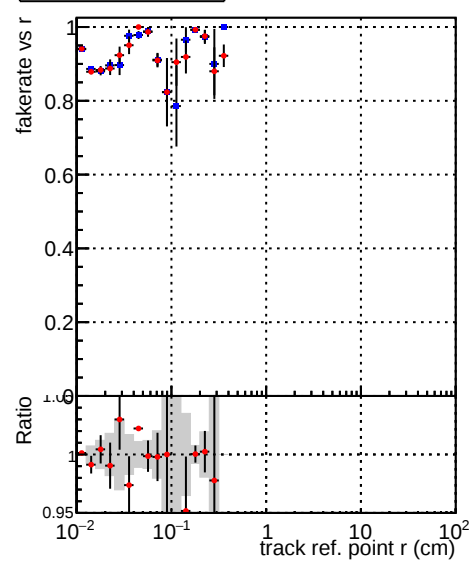
■ DQM_TT_MKFIT_ORIG ● DQM_TT_MKFIT_MODIF
