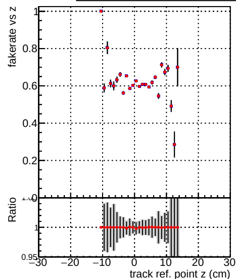
—•— DQM_TT_MKFIT_ORIG —•— DQM_TT_MKFIT_MODIF
