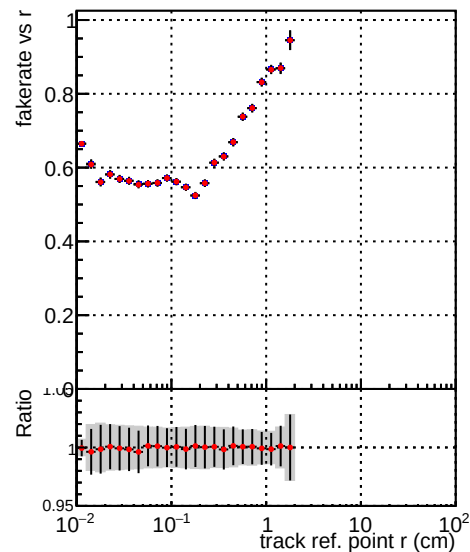
—•— DQM_TT_MKFIT_ORIG —•— DQM_TT_MKFIT_MODIF
