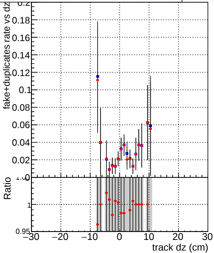
DQM_TT_MKFIT_ORIG DQM_TT_MKFIT_MODIF
