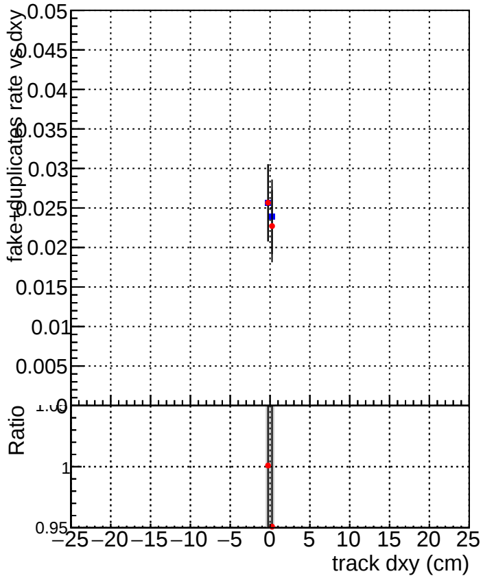
DQM_TT_MKFIT_ORIG DQM_TT_MKFIT_MODIF
