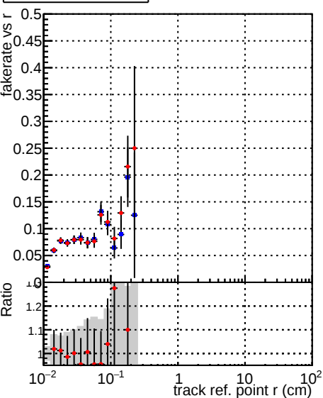
—•— DQM_TT_MKFIT_ORIG —•— DQM_TT_MKFIT_MODIF
