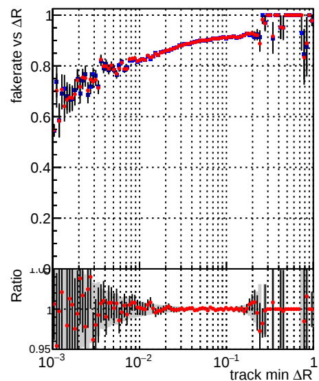
—•— DQM_TT_MKFIT_ORIG —•— DQM_TT_MKFIT_MODIF
