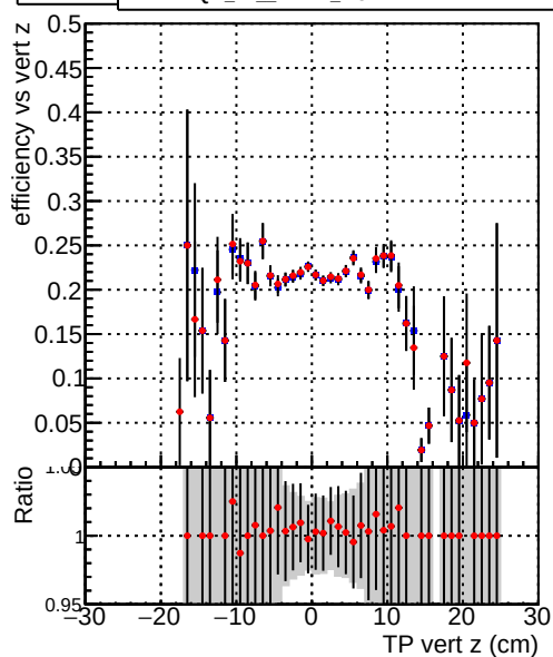
Efficiency vs vert z — DQM_TT_MKFIT_ORIG — DQM_TT_MKFIT_MODIF
