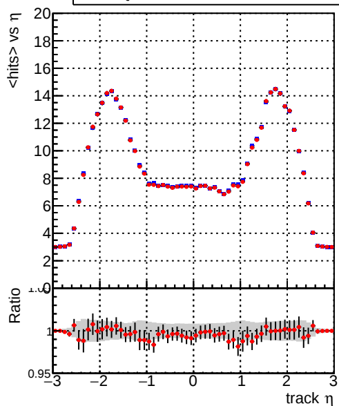
— DQM_TT_MKFIT_ORIG — DQM_TT_MKFIT_MODIF
