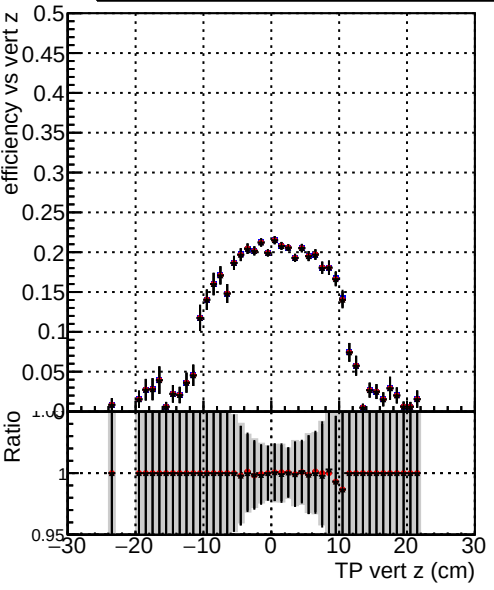
Efficiency vs vertpos DQM_TT_CKF_ORIG DQM_TT_CKFLowPt_ORIG DQM_TT_CKFLowPt_MODIF
