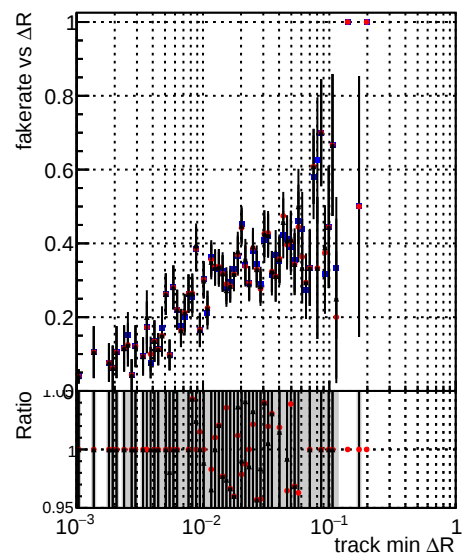
—●— DQM_TT_CKF_ORIG —●— DQM_TT_CKFLOWPtT_ORIG —●— DQM_TT_CKFLOWPtT_MODIF
