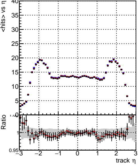
mean hits — DQM_TT_CKFlowPt_ORIG (blue) — DQM_TT_CKFlowPtT_ORIG (red) — DQM_TT_CKFlowPtT_MODIF (black)
