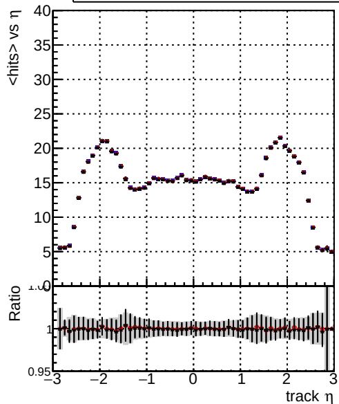
mean hits vs \eta DQM_TT_CKF_ORIG DQM_TT_CKFlowPIT_ORIG DQM_TT_CKFlowPIT_MODIF
