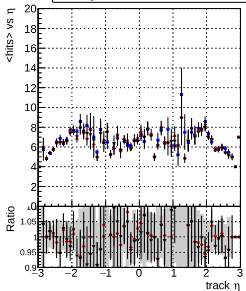
mean hits — DQM_TT_CKF_ORIG — DQM_TT_CKFlowPiT_ORIG — DQM_TT_CKFlowPiT_MODIF
