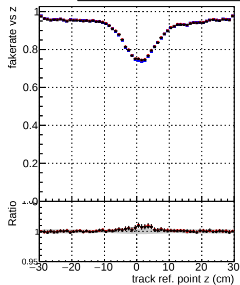
—●— DOM_TT_CKFLowPtT_ORIG —●— DOM_TT_CKFLowPtT_ORIG —●— DQM_TT_CKFLowPtT_MODIF
