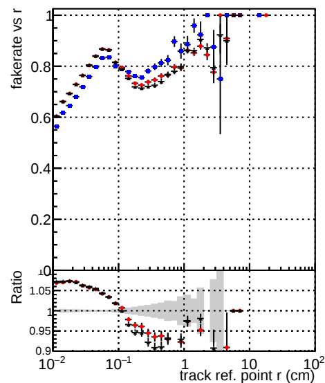
—●— DQM TT CKF ORIG —*— DQM TT CKFLowPtT ORIG —x— DQM TT CKFLowPtT MODIF
