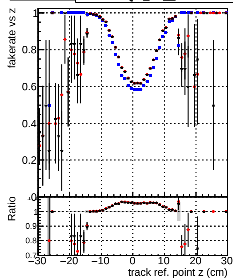
—●— DQM TT CKF ORIG —*— DQM TT CKFLowPtT ORIG —x— DQM TT CKFLowPtT MODIF
