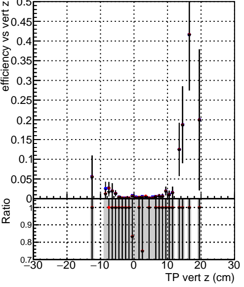
Efficiency vs TP vert z (cm) DQM_TT_CKF_ORIG DQM_TT_CKFLowPtT_ORIG DQM_TT_CKFLowPtT_MODIF
